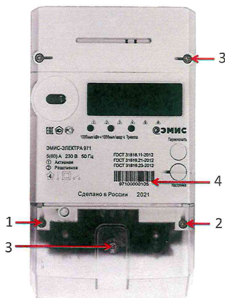
Рисунок 3 – Общий вид счетчика исполнения «Х» со схемой пломбировки
